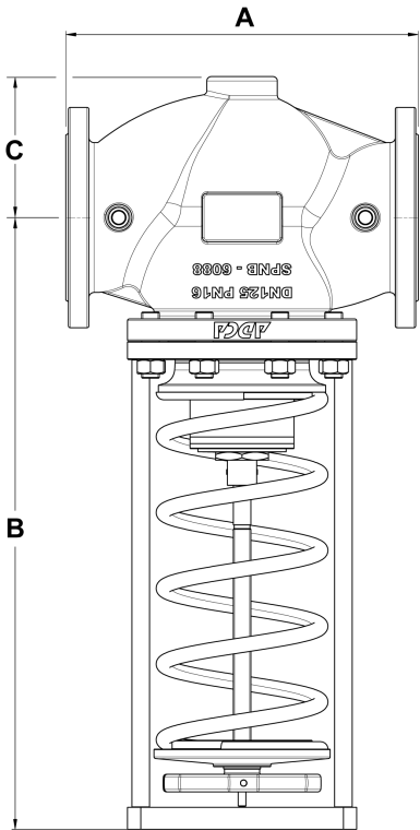
DN 125 bis DN 150
