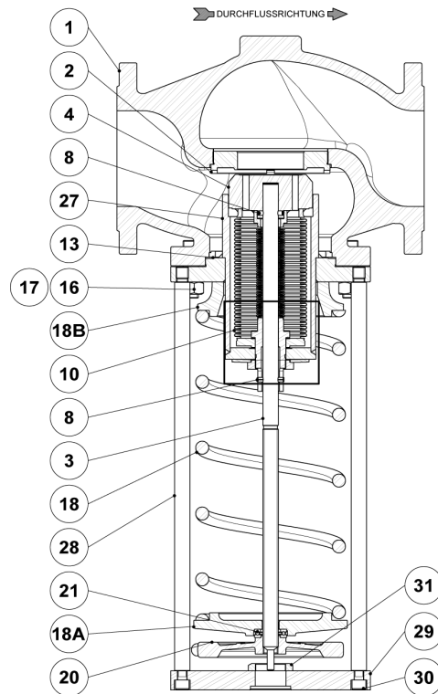
DN 125 bis DN 150
