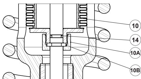
Detailansicht B (DN 80 und DN 100)
