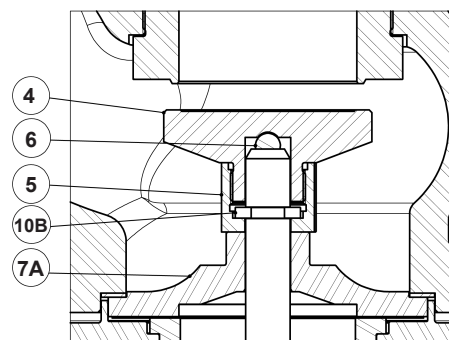
Detailansicht A (DN 80 und DN 100)
