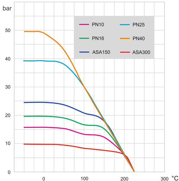
Gehäuse A216 WCB / Metall-Metall Sitz
