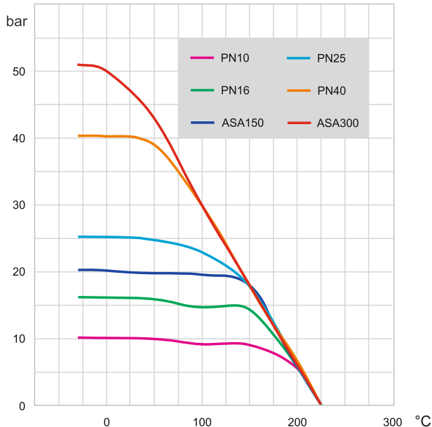
Gehäuse A216 WCB / PTFE Sitz
