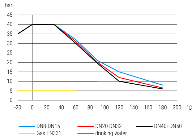
Druck-Temperatur-Diagramm pressure-temperature-diagram
