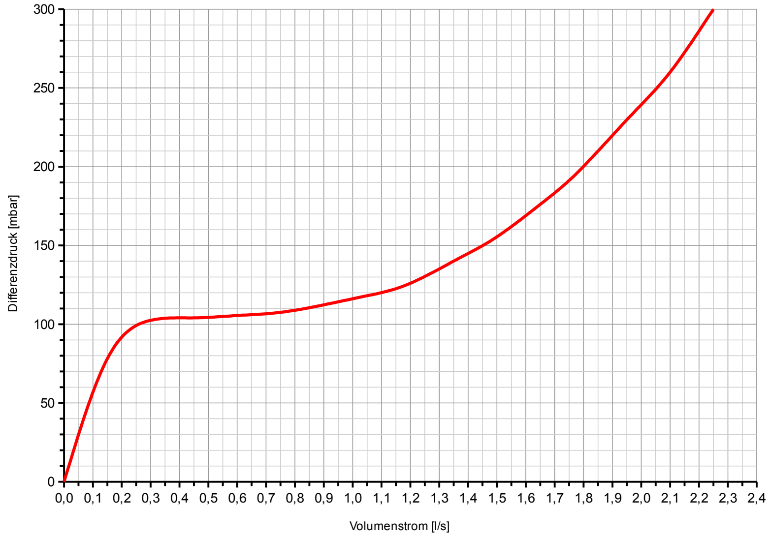
Differenzdruckmessung DN25
